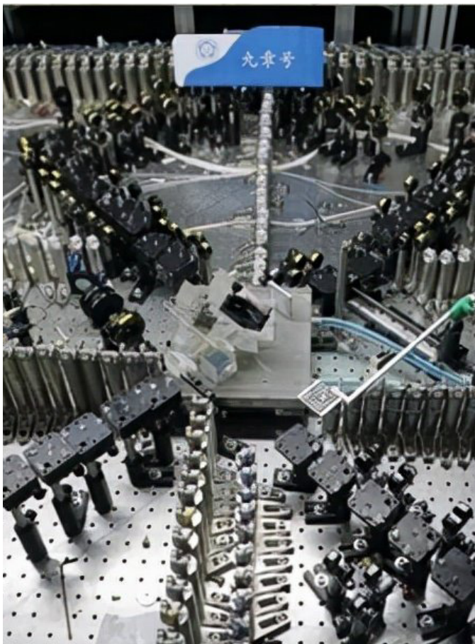
Le prototype d'ordinateur quantique optique « Jiuzhang 2.0 ».
